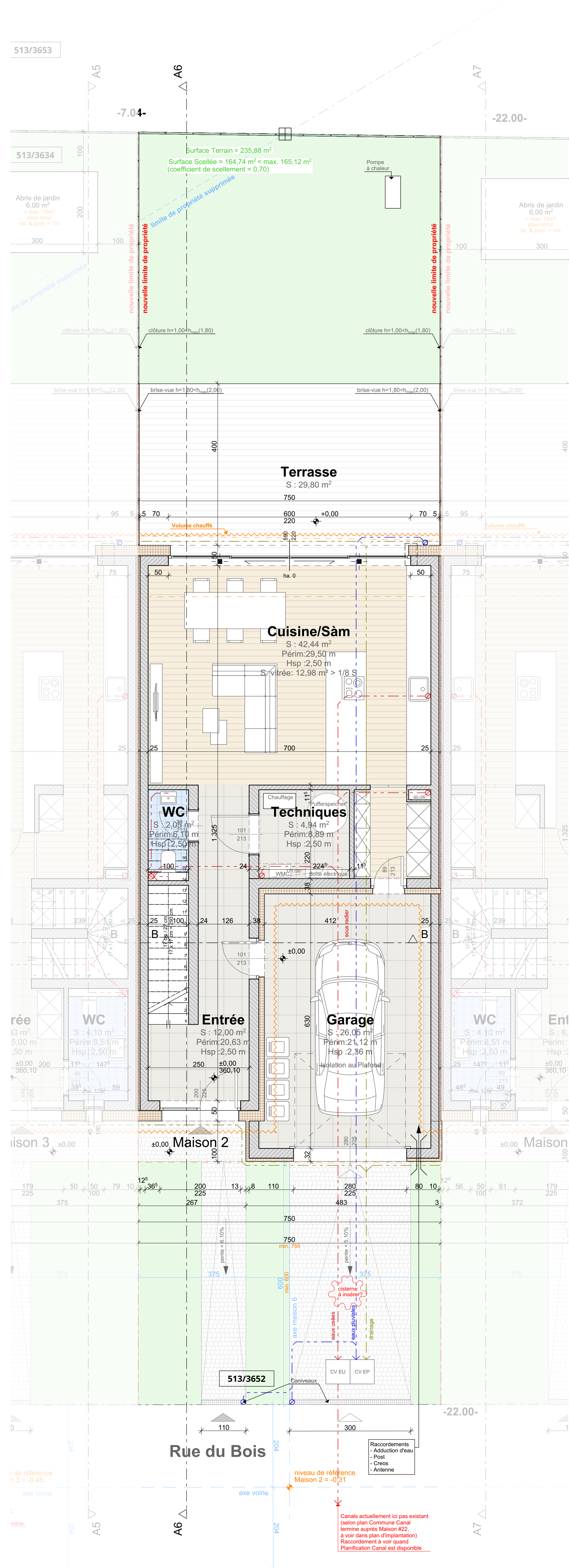
0. Rez-de-chaussée 1:50
