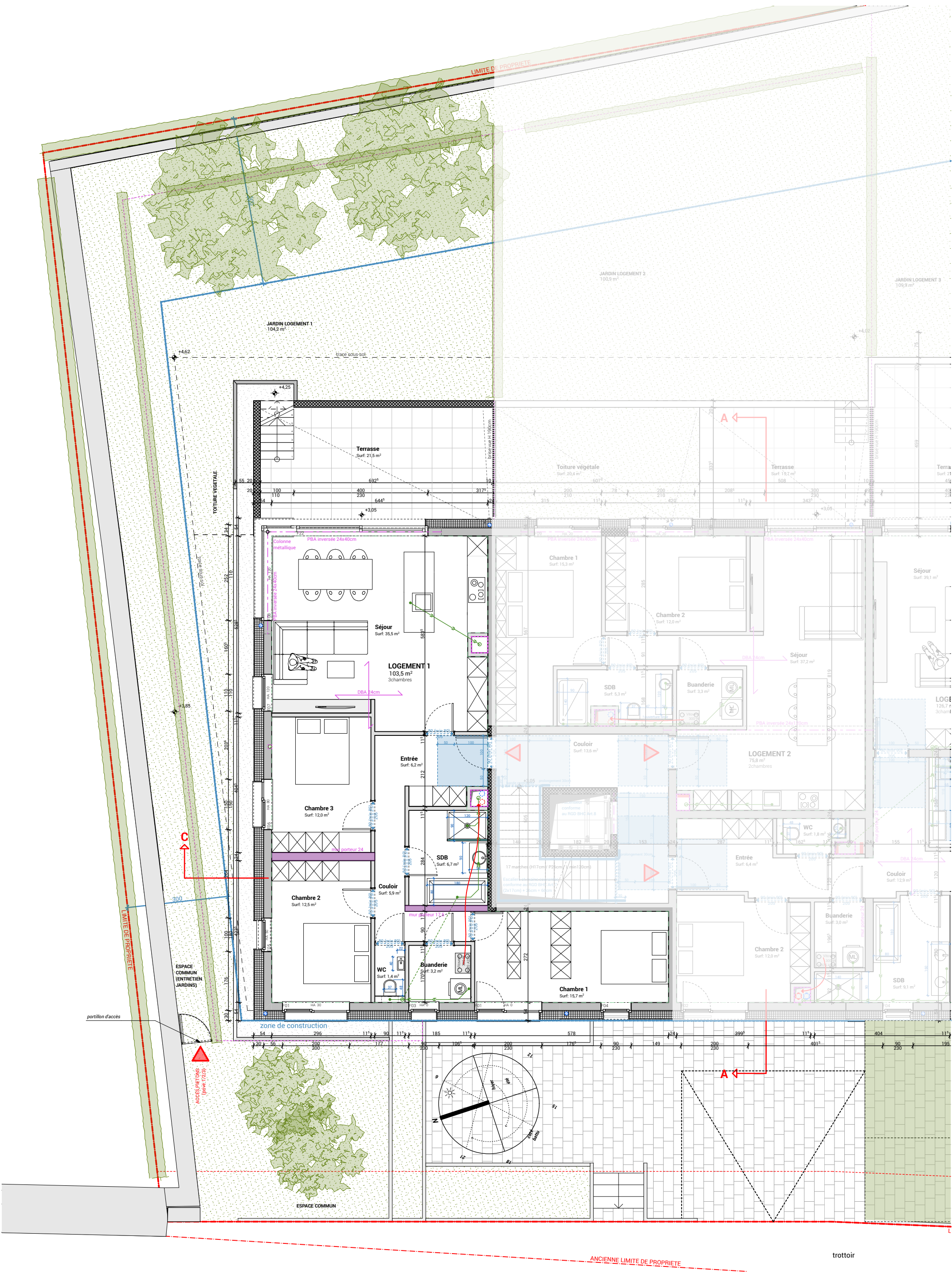
Plan Etage 1 (niveau jardin)
